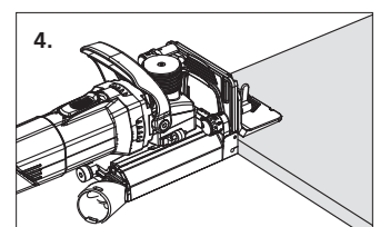
4. Mit positionierter Maschine fräsen
