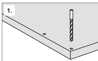
1. Positionsbohrung mit CNC, Ø 5 mm / Ø 8 mm
