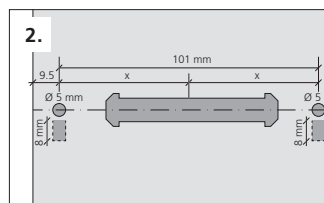
2. Bohrbild der Positionierbohrungen
