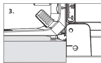
3. Positionierclip in Bohrung Ø 6 mm stecken
