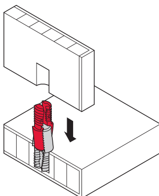
1. Verbinder in die Bohrung einpressen
