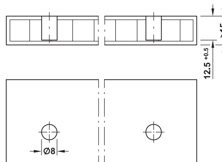
Bohrung in der Fläche
