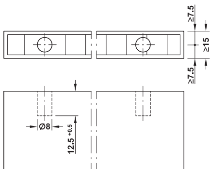
stirnseitige Bohrung
