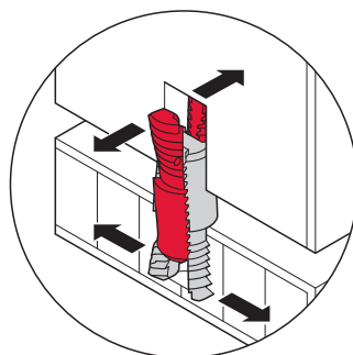
2. beide Plattenteile zusammenstecken; die beiden Verbinderteile verspreizen sich synchron in der Bohrung
